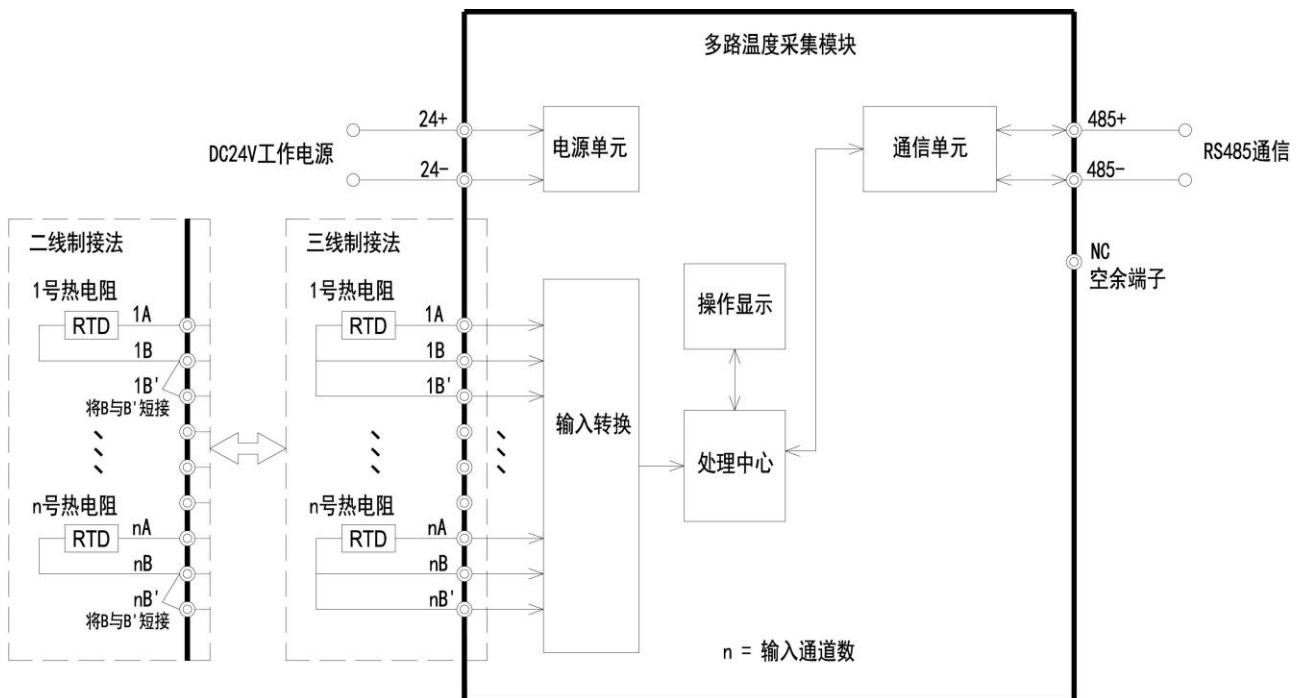
信号输入接线示意图:
